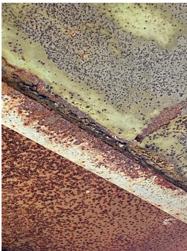
Фото №19-21. Коррозионные повреждения верхних полок двутавров обвязки верхней площадки.
